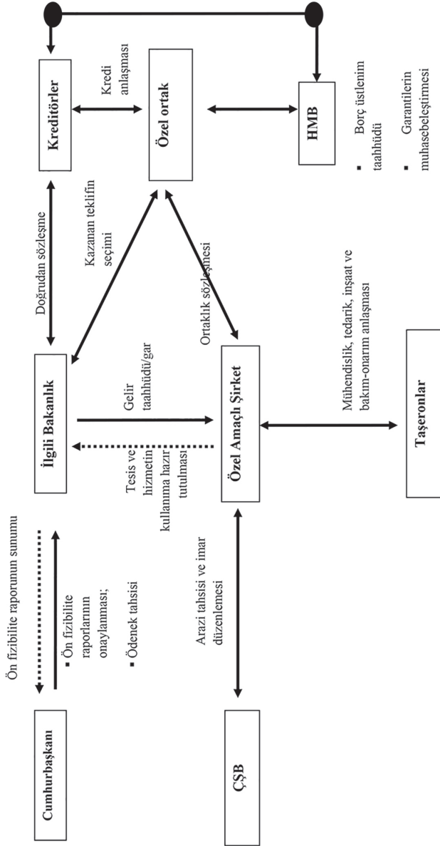
Şekil 12. Kurumsal yapı
